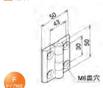
9 蝶番
